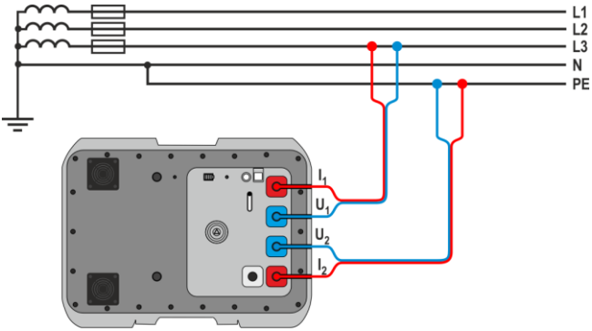
Medición de la impedancia en el circuito de protección (L-PE).
