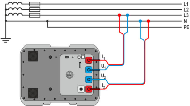
Medición de la impedancia en el circuito de trabajo (L-N).
