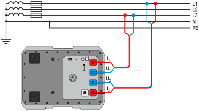
Medición de la impedancia en el circuito de trabajo (L-L).
